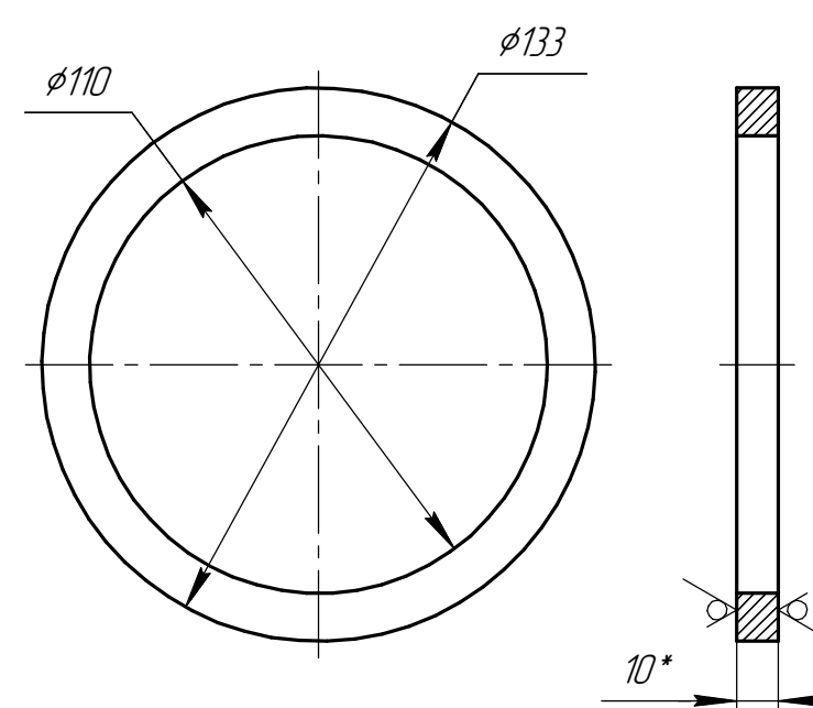
Дет. поз. 3
